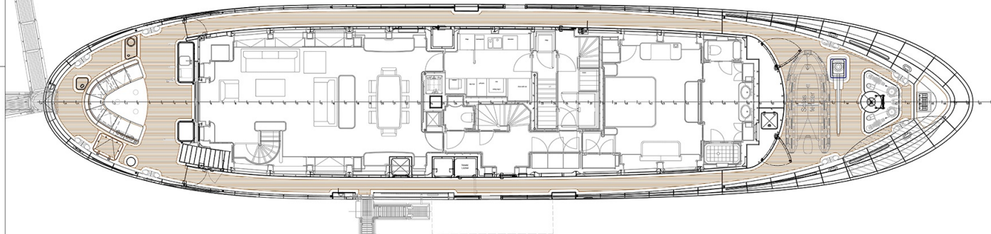
CABINDECK
