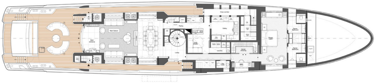
PONTE COPERTA / MAIN DECK
