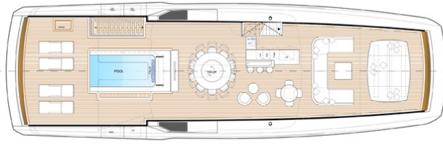
PONTE SOLE / SUN DECK
