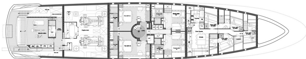
PONTE SOTTOCOPERTA / LOWER DECK
